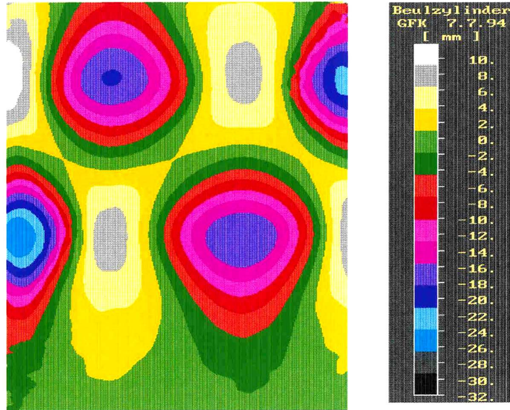
Beulmuster eines GFK-Zylinders unter axialer Last
