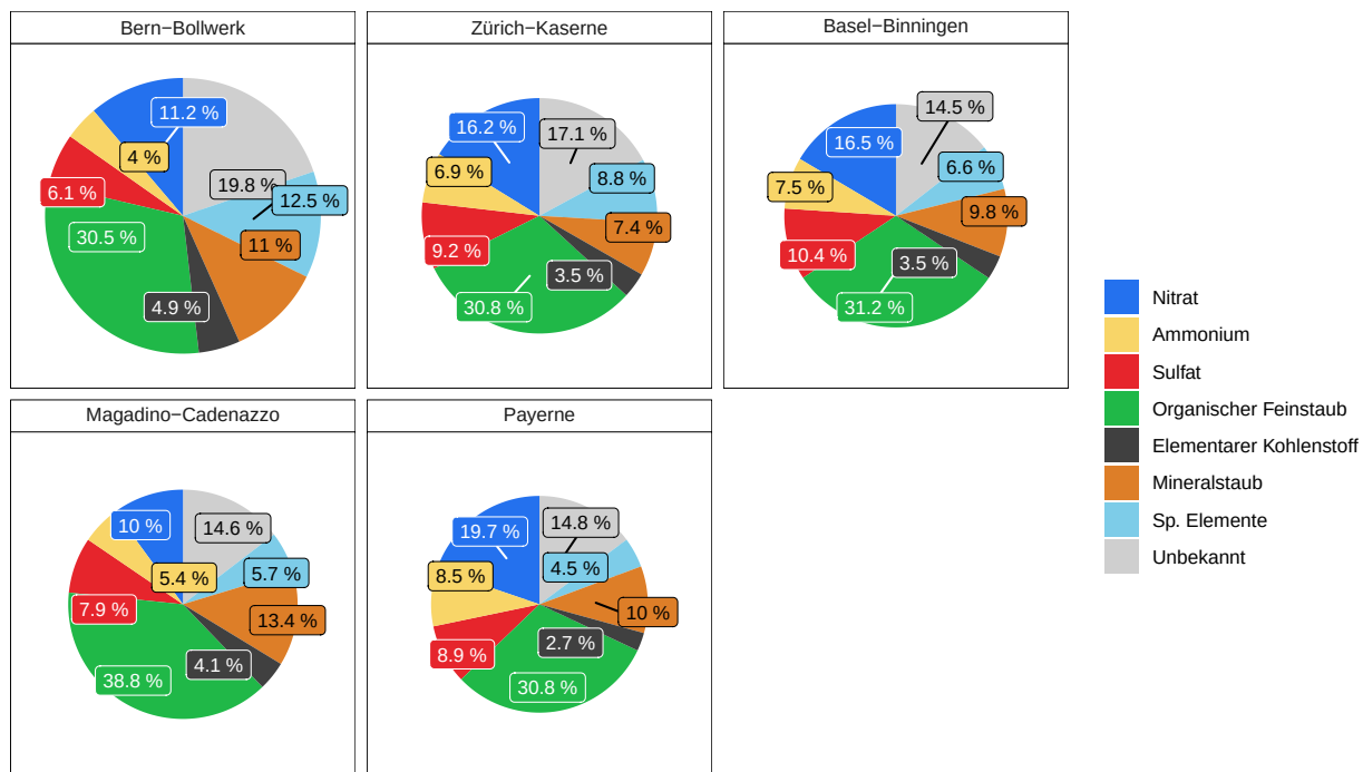
Abbildung 1: Mittlere chemische Zusammensetzung von PM_{10} an den fünf Messstationen der Messkampagne von 2018–2019. Die Fläche der Kreise ist proportional zur gesamten Konzentration von PM_{10} an den unterschiedlichen Standorten (Bern-Bollwerk: 21.3 \mu g m^{-3} , Zürich-Kaserne: 15.6 \mu g m^{-3} , Basel-Binningen: 14.0 \mu g m^{-3} , Magadino-Cadenazzo: 14.8 \mu g m^{-3} , Payerne: 13.2 \mu g m^{-3} ).
