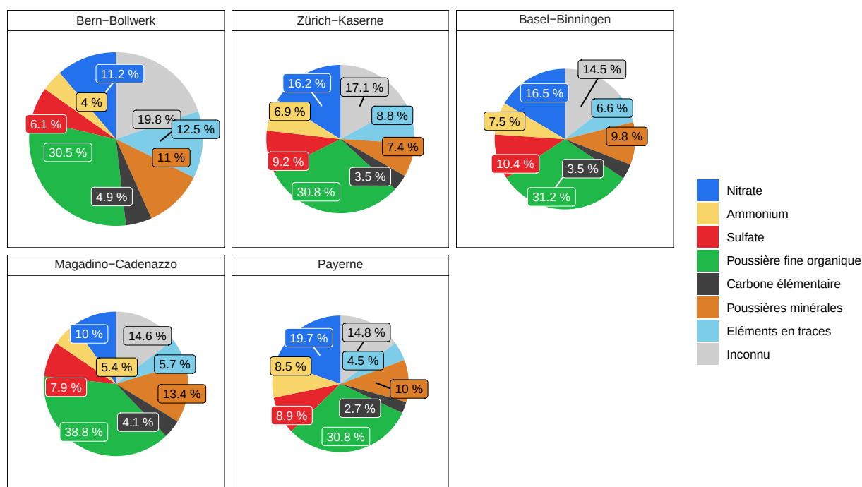
Figure 1 : Composition chimique moyenne des PM 10 mesurée sur les cinq sites de la campagne 2018-2019. La surface des cercles est proportionnelle à la concentration totale en PM 10 relevée sur chaque site (Bern-Bollwerk : 21.3 µg m -3 , Zürich-Kaserne : 15.6 µg m -3 , Basel-Binningen : 14.0 µg m -3 , Magadino-Cadenazzo : 14.8 µg m -3 , Payerne : 13.2 µg m -3 ).
