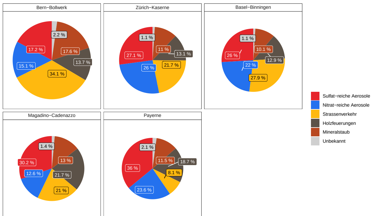
Abbildung 4: Mittlere Beiträge der mit einem statistischen Modell bestimmten Quellen von \text{PM}_{10} an den fünf Messstationen der Messkampagne von 2018–2019. Die Fläche der Kreise ist proportional zur gesamten Konzentration von \text{PM}_{10} an den unterschiedlichen Standorten (Bern-Bollwerk: 21.3 \mu\text{g m}^{-3} , Zürich-Kaserne: 15.6 \mu\text{g m}^{-3} , Basel-Binningen: 14.0 \mu\text{g m}^{-3} , Magadino-Cadenazzo: 14.8 \mu\text{g m}^{-3} , Payerne: 13.2 \mu\text{g m}^{-3} ).
