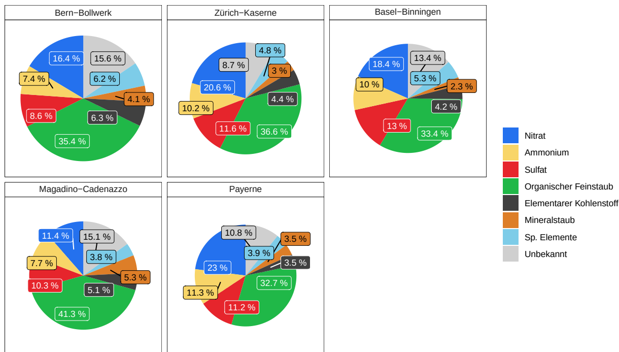
Abbildung 2: Mittlere chemische Zusammensetzung von PM_{2.5} an den fünf Messstationen der Messkampagne von 2018–2019. Die Fläche der Kreise ist proportional zur gesamten Konzentration von PM_{2.5} an den unterschiedlichen Standorten. (Bern-Bollwerk: 14.0 \mu g m^{-3} , Zürich-Kaserne: 11.1 \mu g m^{-3} , Basel-Binningen: 10.6 \mu g m^{-3} , Magadino-Cadenazzo: 10.4 \mu g m^{-3} , Payerne: 9.2 \mu g m^{-3} ).
