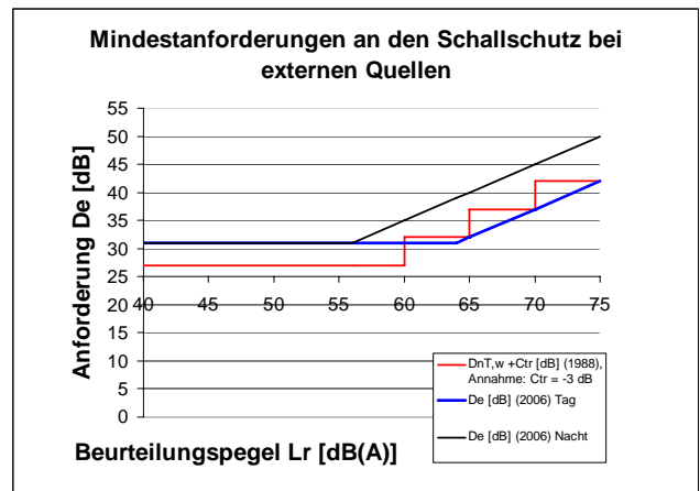
Abbildung 2: Vergleich der Anforderungen gegen Luftschall von aussen nach Norm SIA 181 (1988, rot) und nach Norm SIA 181 (2006, schwarz bzw. blau), jeweils für Lärmempfindlichkeit „mittel“
