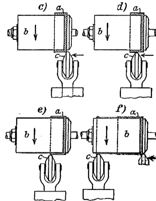
Abb. 280. Drücken von gegossenen Gefäßen (Verfahren Kuhn).
